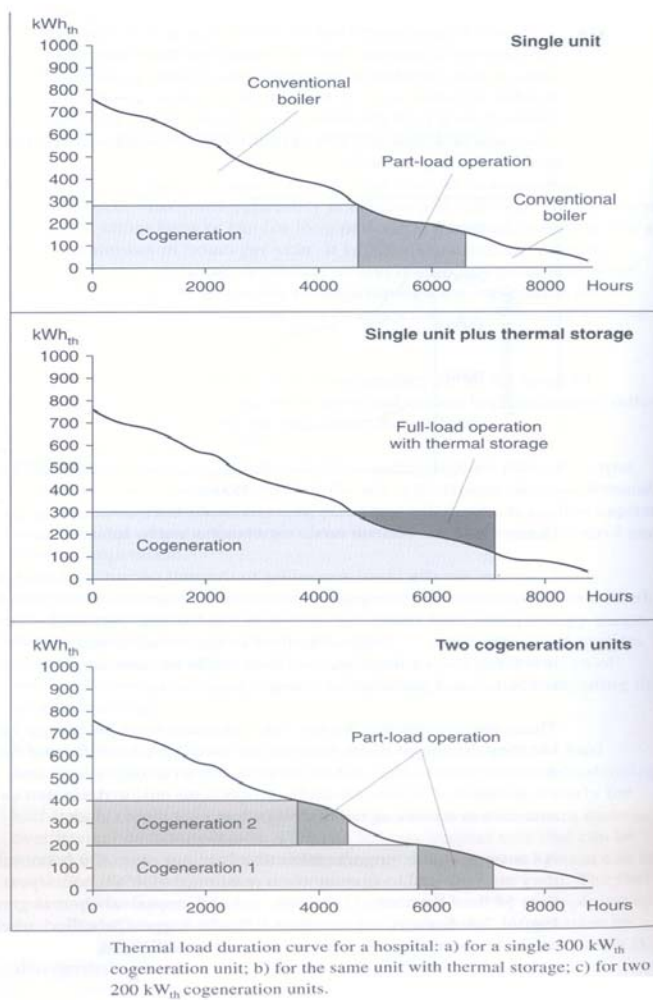
شکل ۸- مقایسه تولید مشترک برق و حرارت در حالت‌های مختلف در یک بیمارستان
